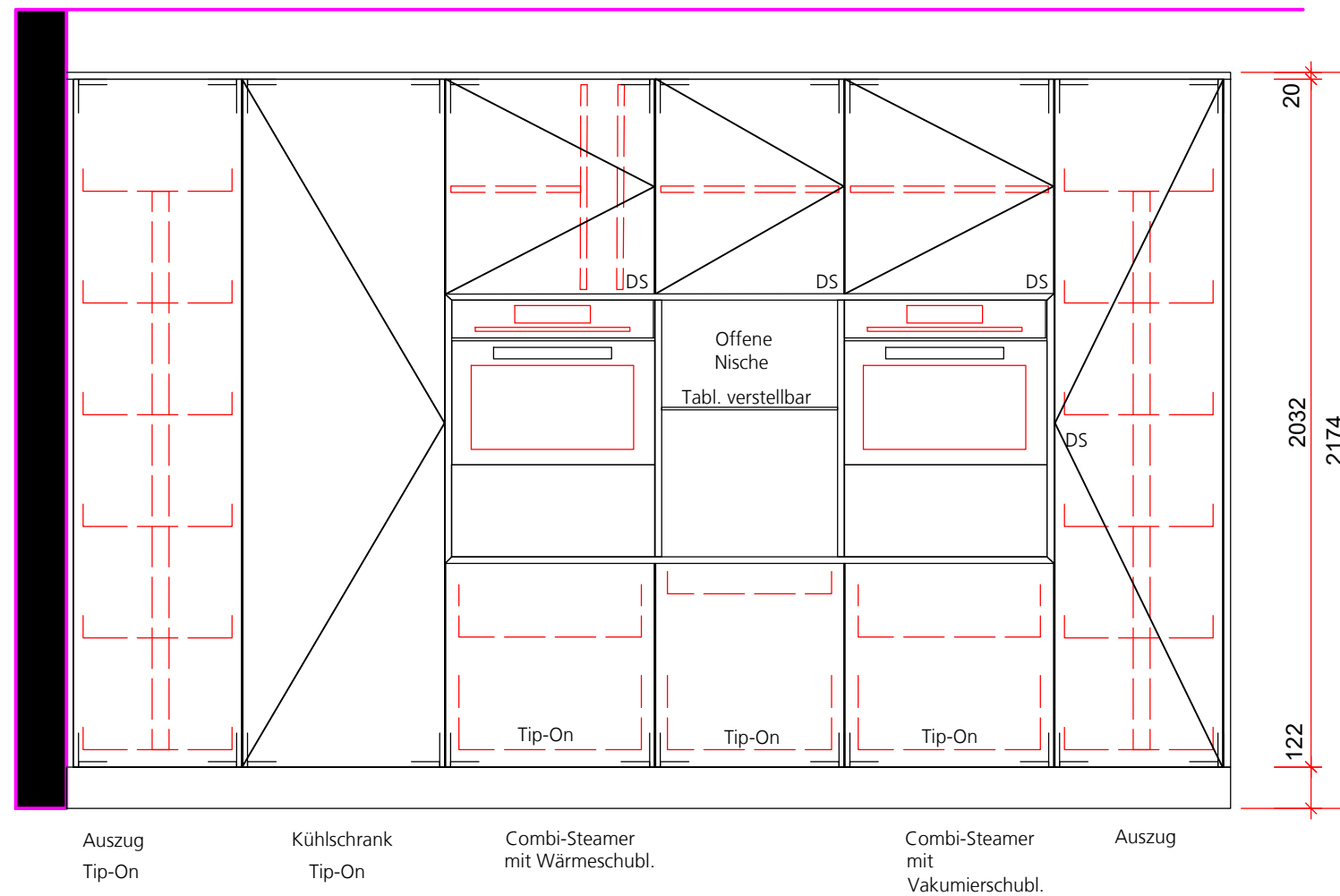
Ansicht A
