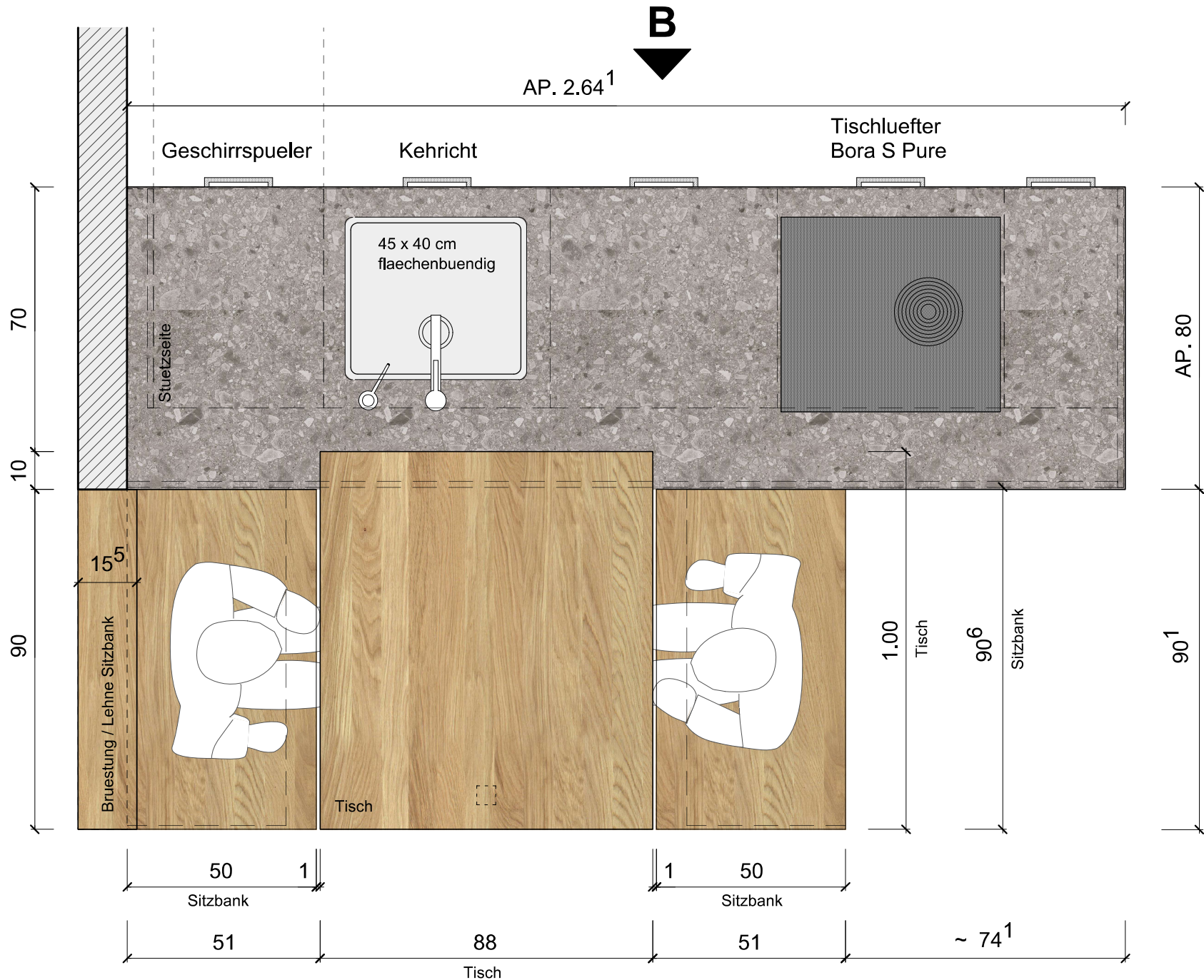
Grundriss Insel
