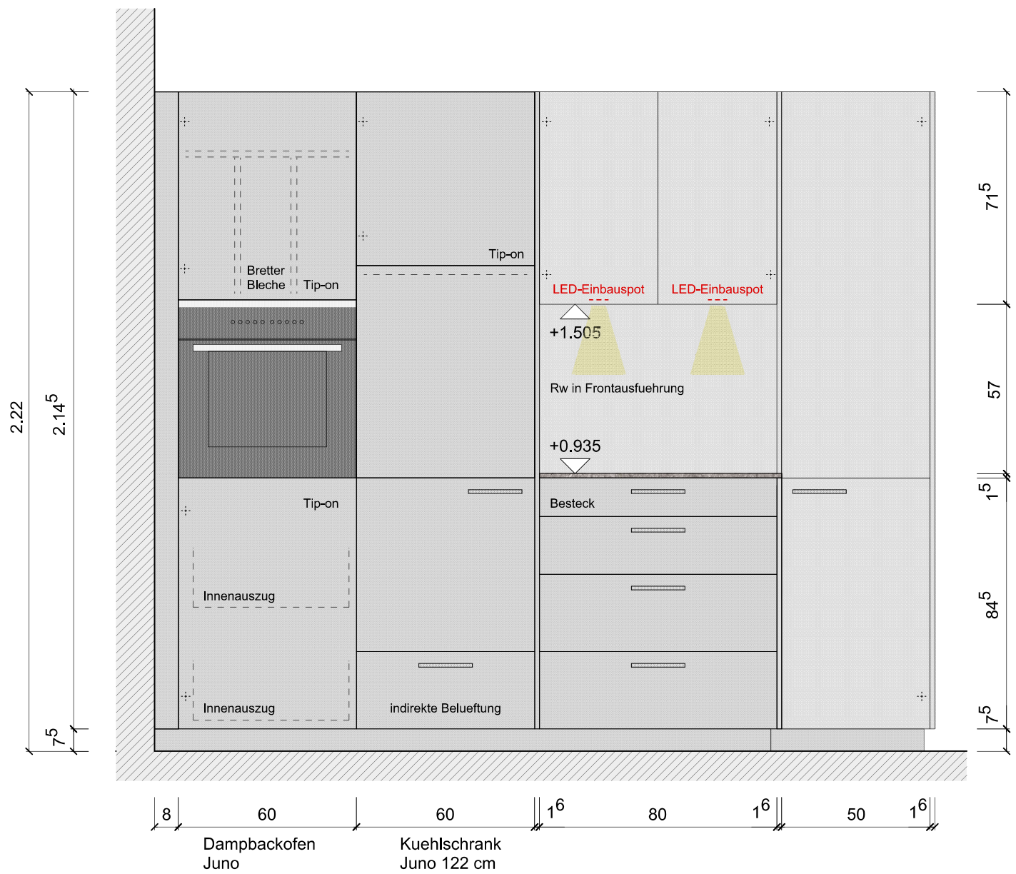
Ansicht A Hochschrankanlage
