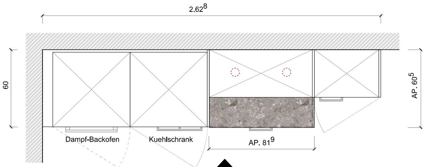
Grundriss Hochschrankanlage
