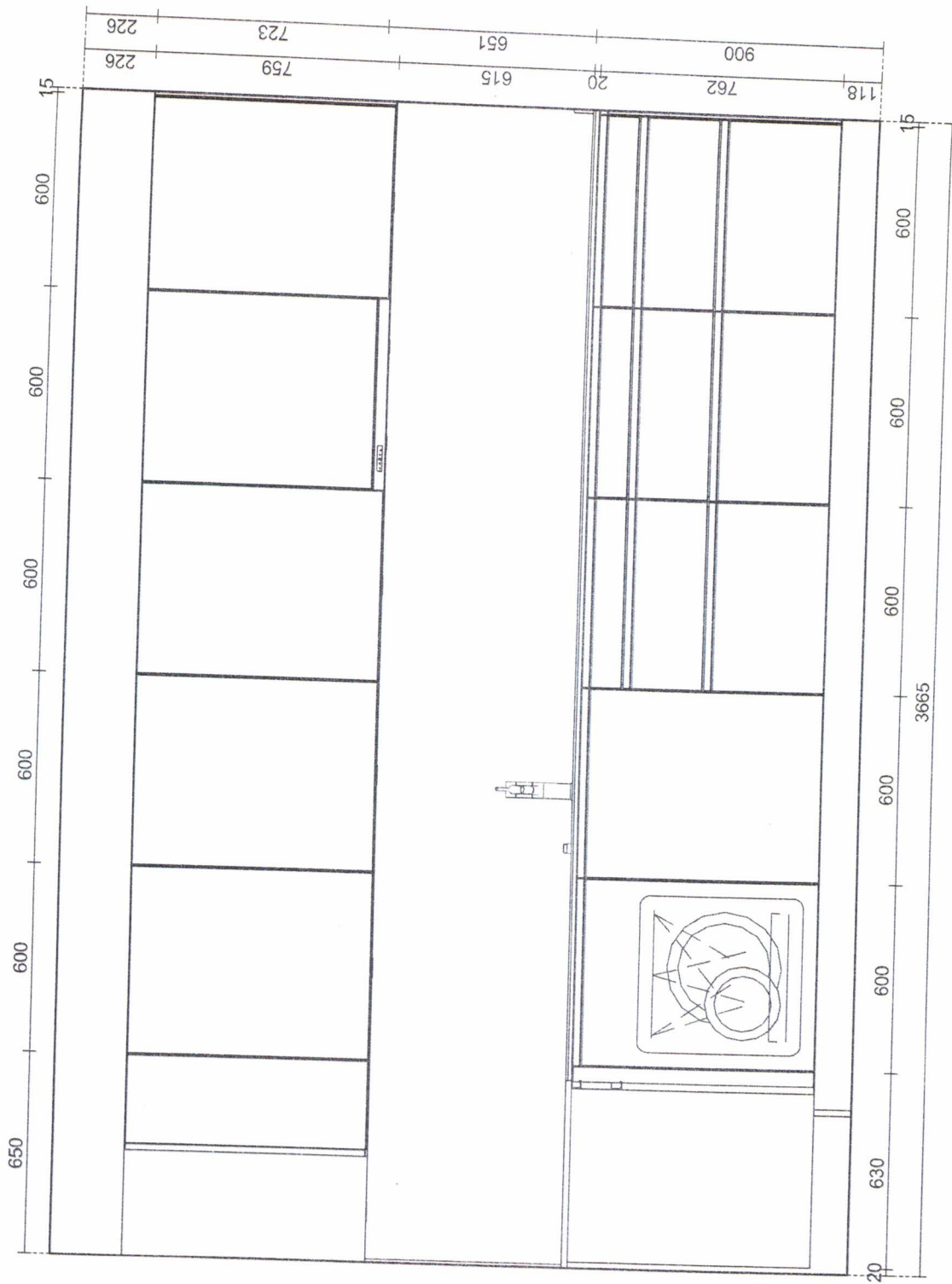
Wand - 3 / Massstab: 1:20 (A4)
